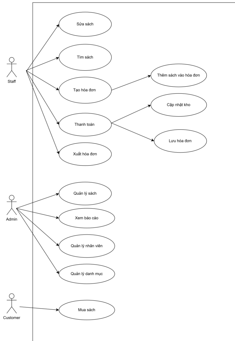
Hình 1. Mô tả Use Case
